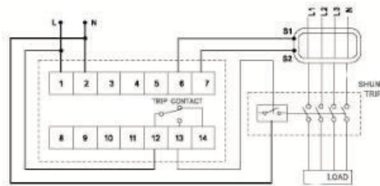
Τυπικό σχέδιο εφαρμογής KLR523
